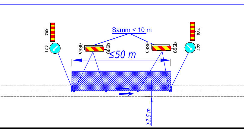
Töömaa tähistamise tüüpskeem
